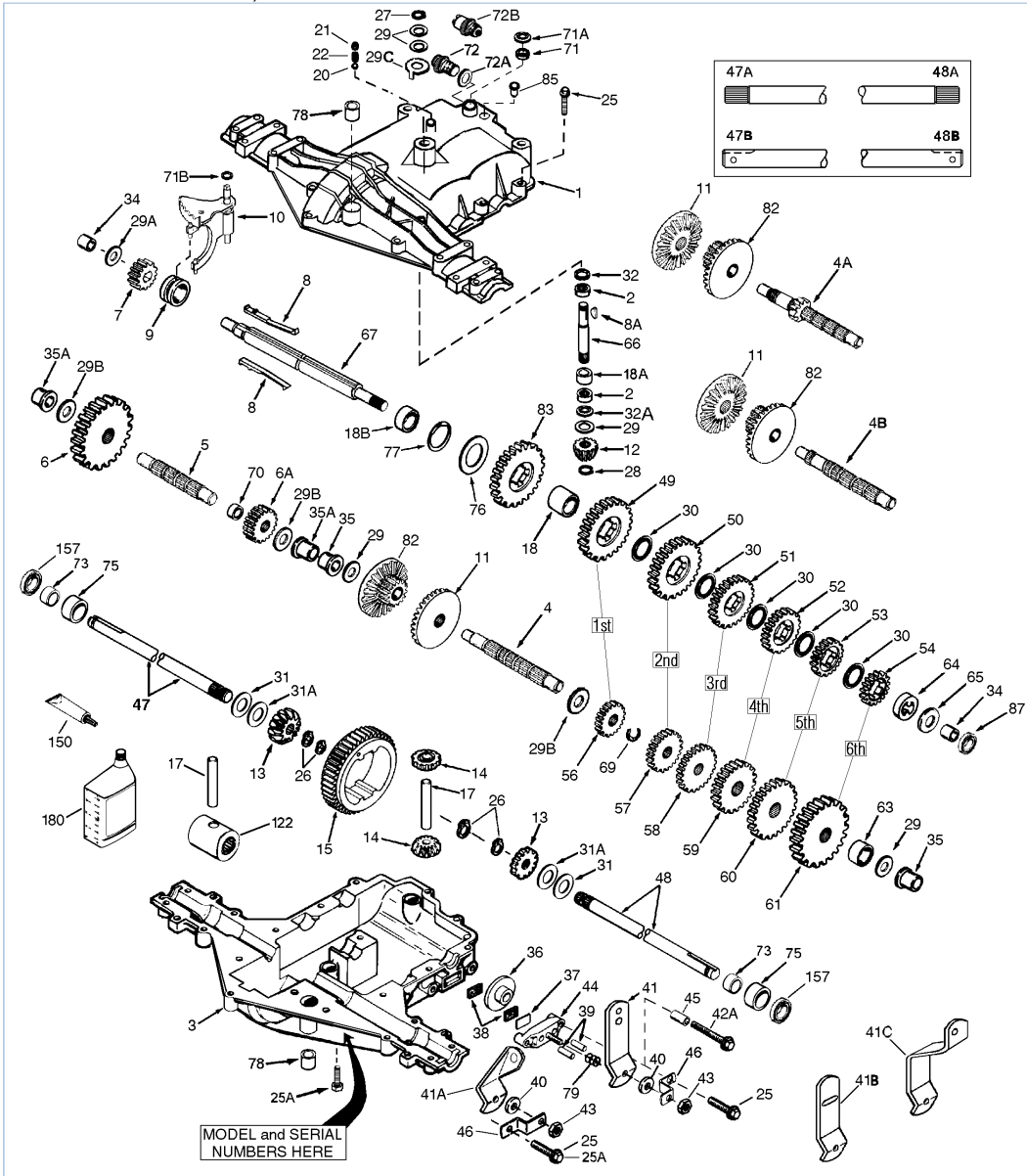
mst.2 206-206-505B / Transaxle
